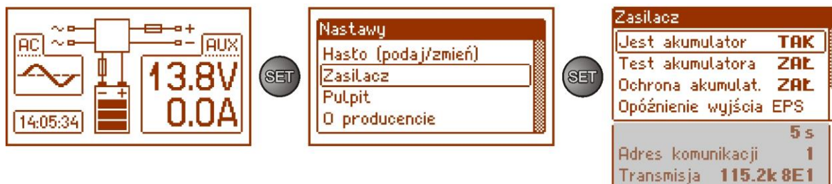
Rys. 22. Ekran „Zasilacz”.
